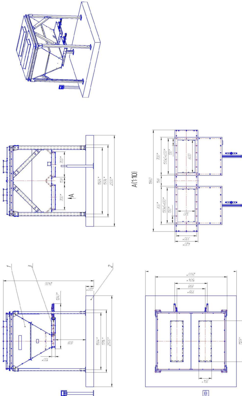
Рис.1 – Дозатор Р1-БДУ-10.00.000 1-бункер; 2- весы платформенные электронные ВПП-2-1; 3-задвижка шибберная с пневмоприводом
